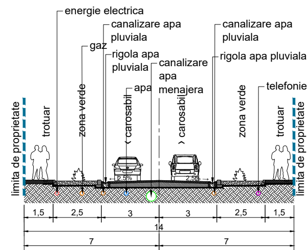
Profil transversal 2-2
