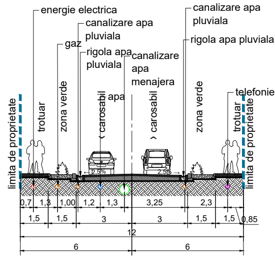
Profil transversal 1-1
